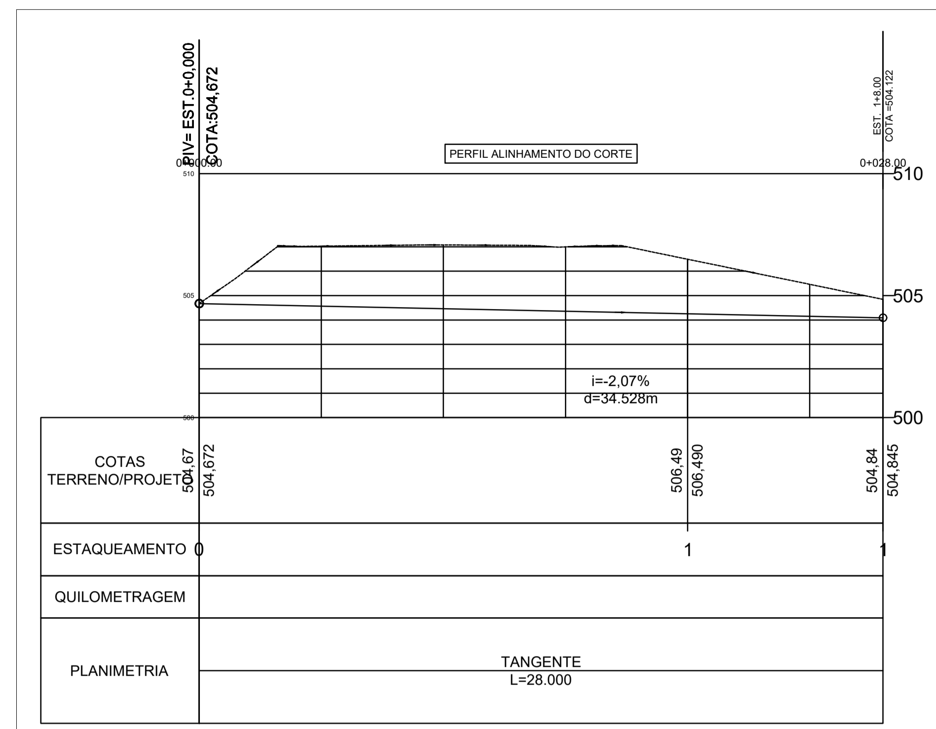
Corte Longitudinal
