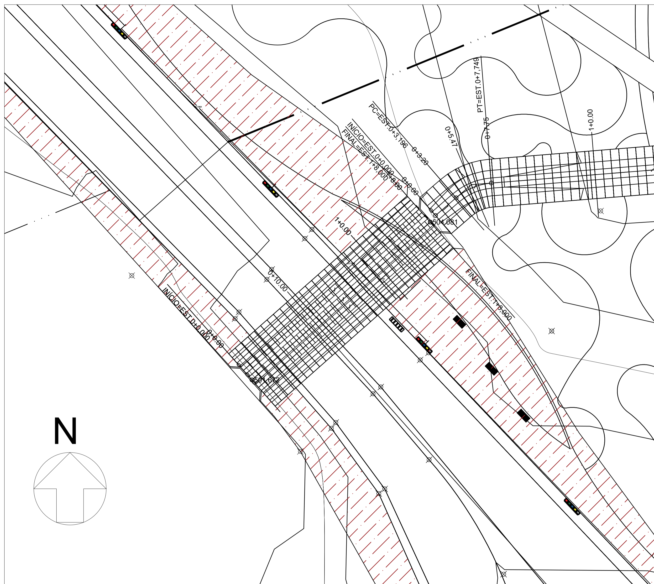
Planta Baixa de Corte para implantação dos Boeiros
