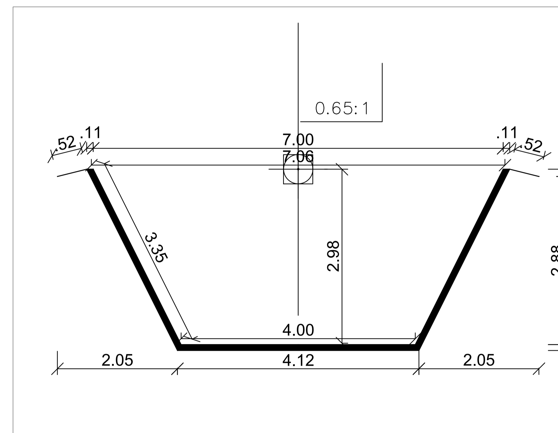
Corte Transversal
